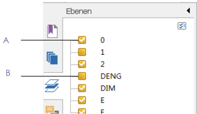
Das Ebenenfenster
